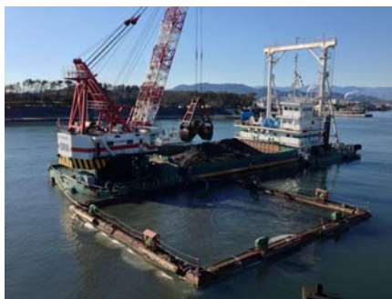
浚渫工事
