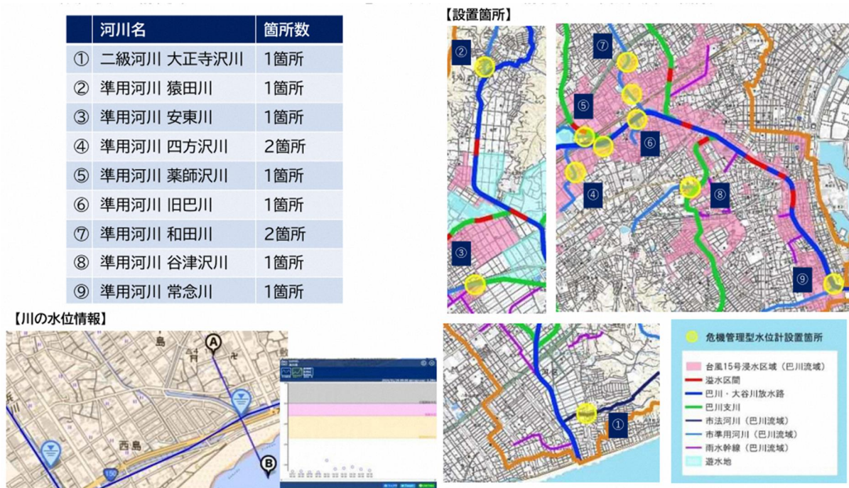
図 5.13 危機管理型水位計の設置箇所（静岡市設置）
