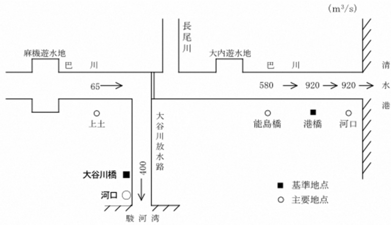
图 5.5 流量配分图
