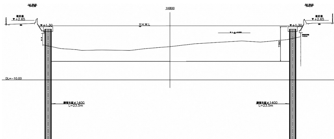
图 5.7 標準断面图
