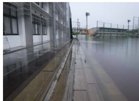
雨水貯留浸透施設の状況 (清水桜が丘高校 令和元年5月撮影)
