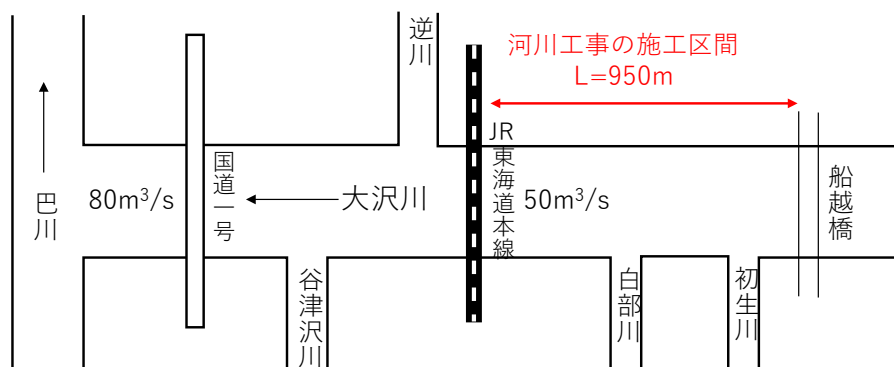
図 4-14 流量配分図
