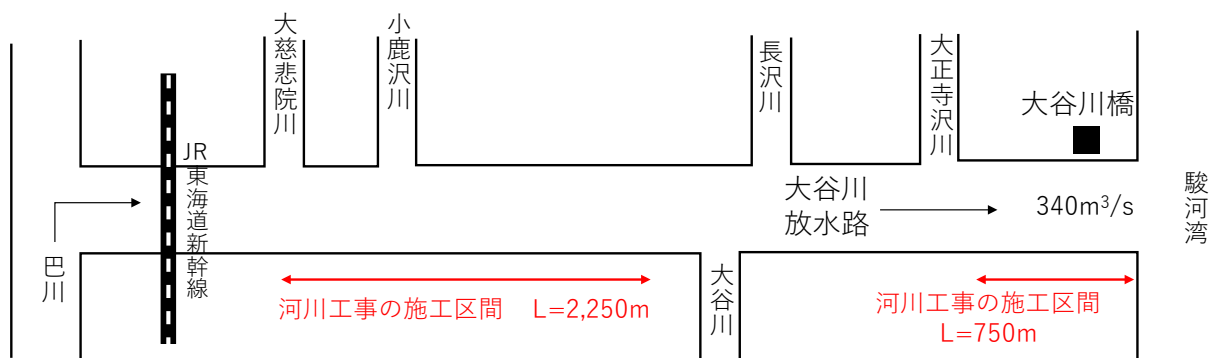
図 4-11 流量配分図
