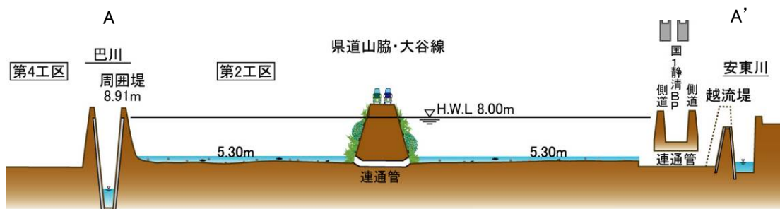
図 4-5 麻機遊水地第2工区横断イメージ図
