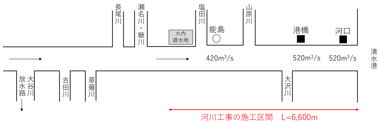
図 4-7 流量配分図
