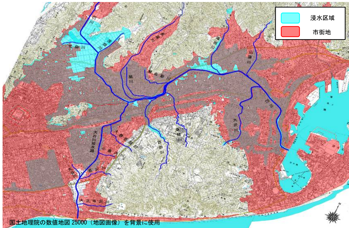
図 2-5 七夕豪雨の浸水エリア (背景は現在の土地利用)
