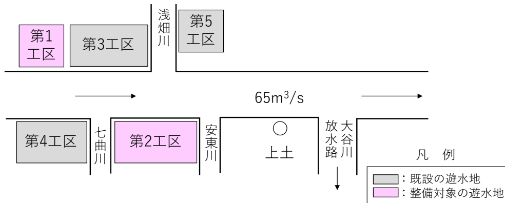
図 4-3 流量配分図
