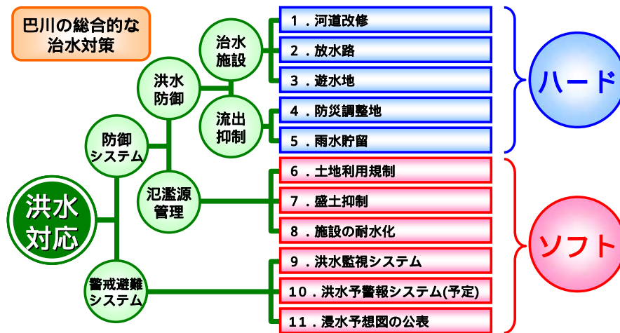
図 2-6 総合的な治水対策システム
