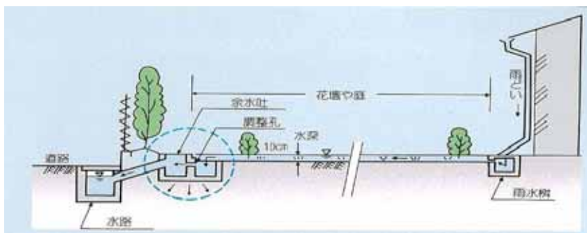
図 2-14 各戸貯留施設の設置状況 -清水区岡町-
