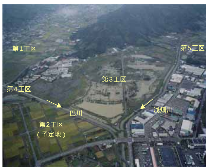
麻機遊水地による洪水調節の状況
