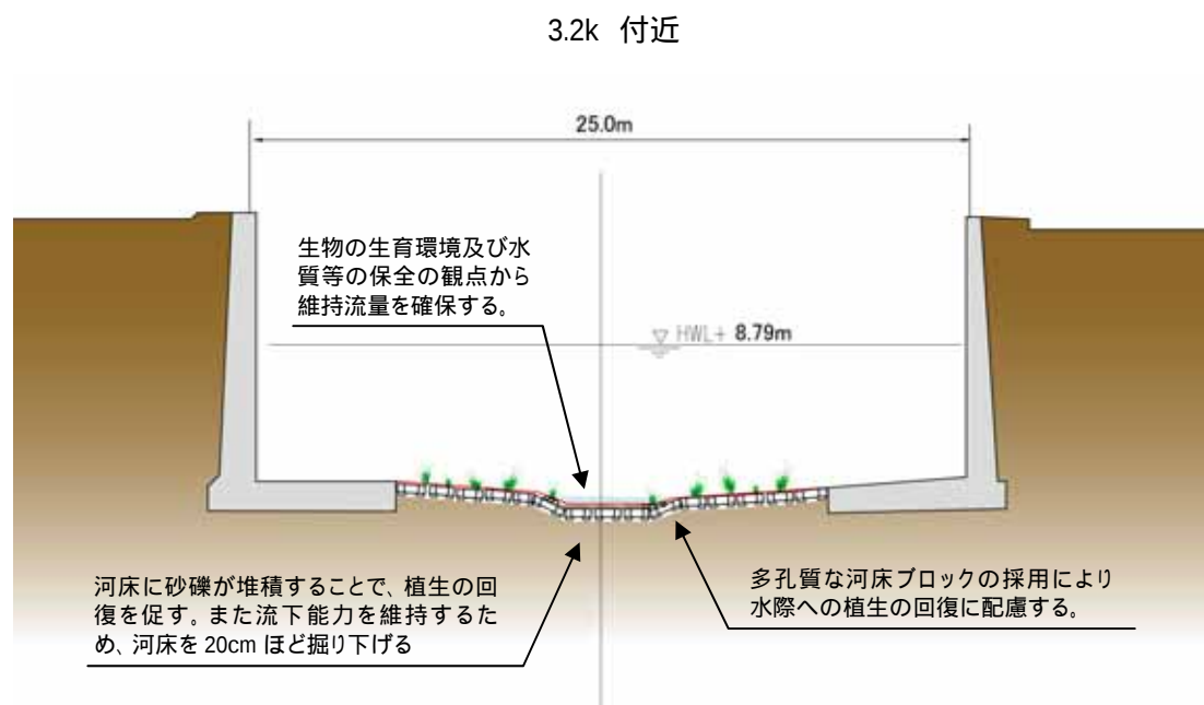
図 4-10 改修横断イメージ図
