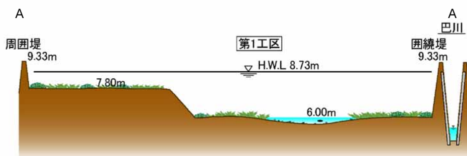
図 4-5 第1工区横断イメージ図
