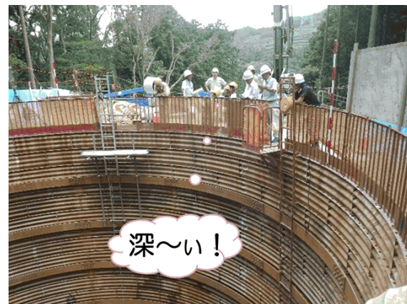
3号橋P5橋脚の深礎杭を見学
