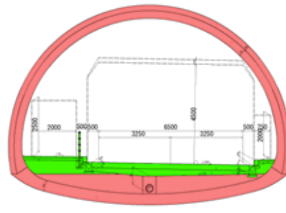
トンネル横断面図
