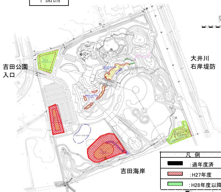
平面図
