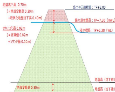
標準横断面図
