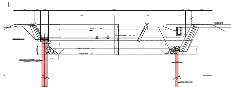
横断面図
