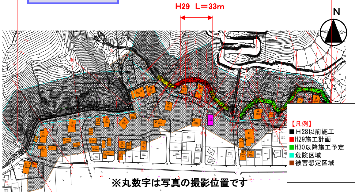
計画平面図
