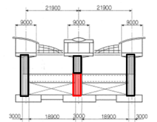
正面図
