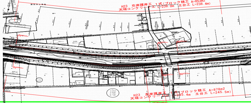
平面図
