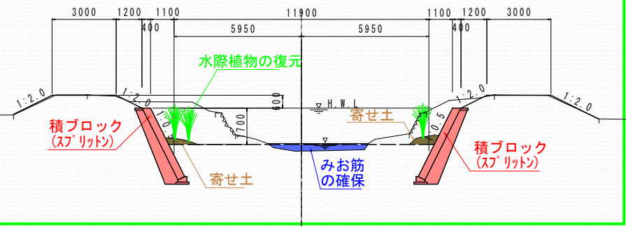
断面図(一般部)
