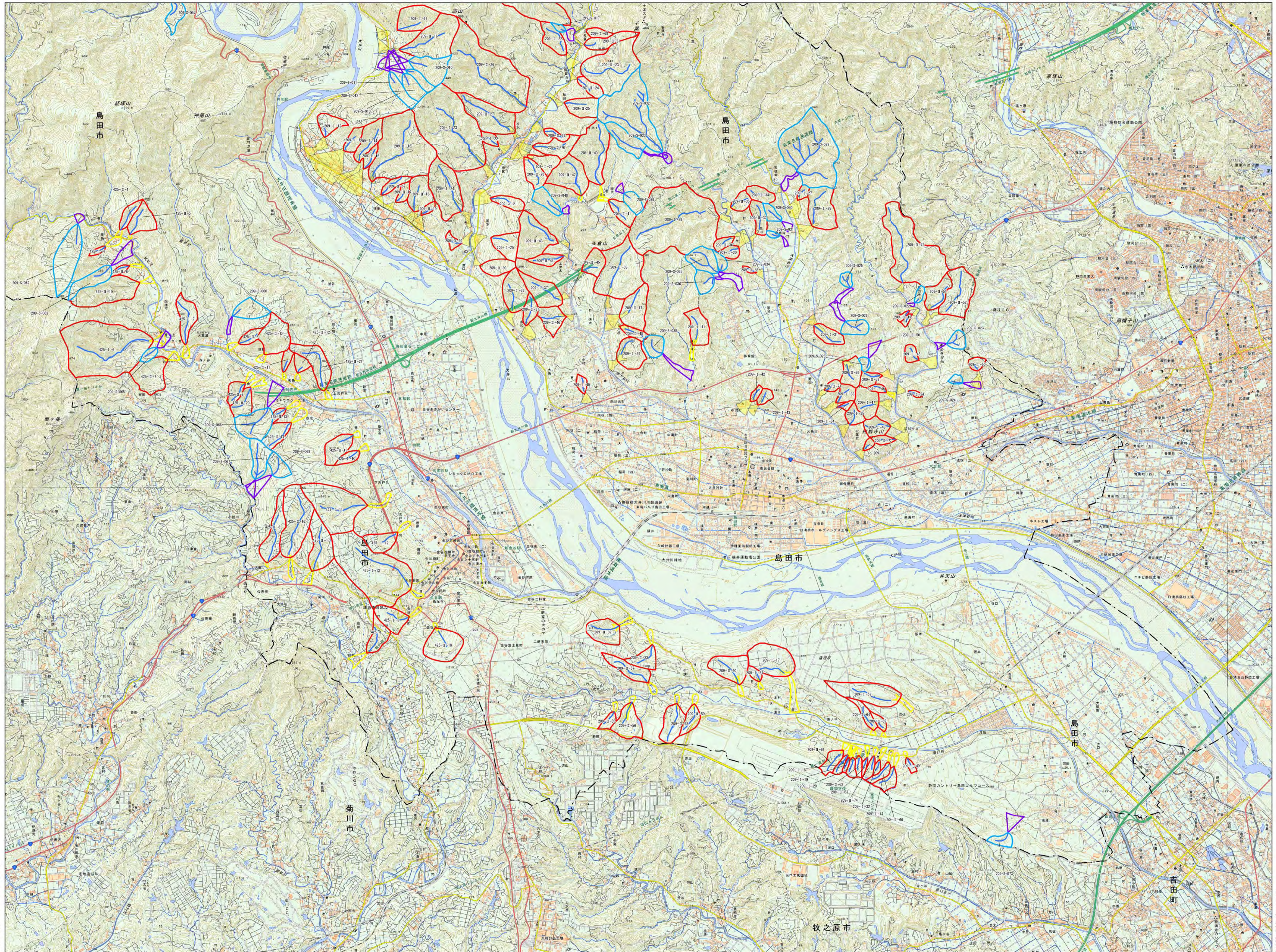
土石流抽出結果平面図 3/3 (島田市)
