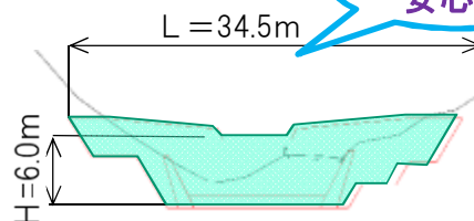
計画施工図
