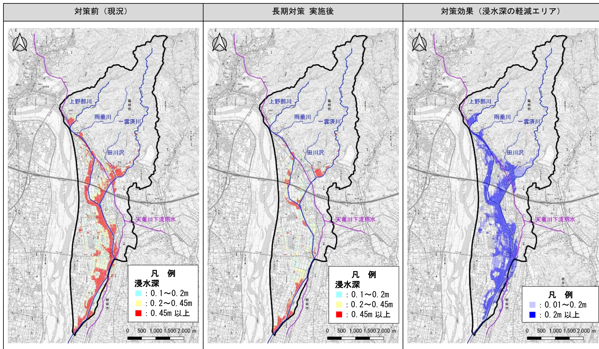
図 5.6 河川対策と流域対策によるシミュレーション結果（長期対策）
