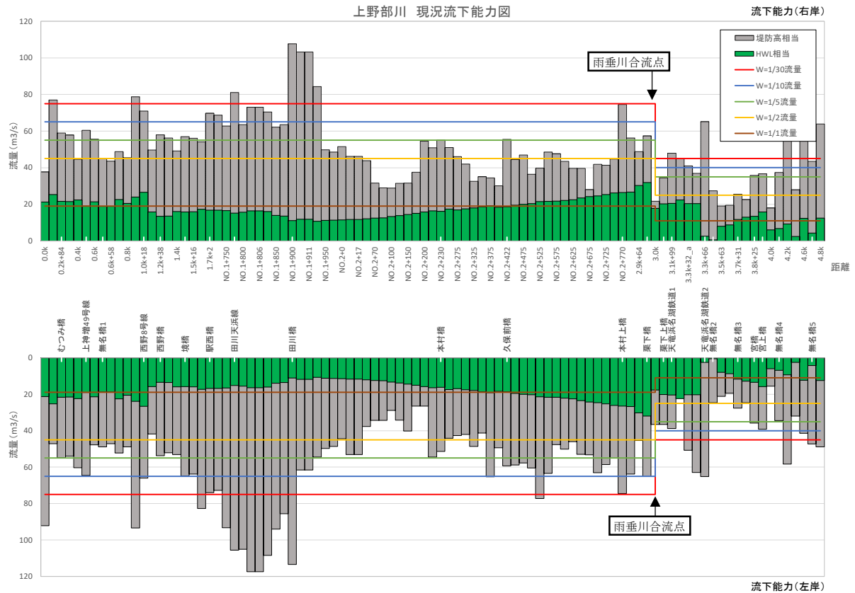
図 3.4 流下能力図（上野部川）
