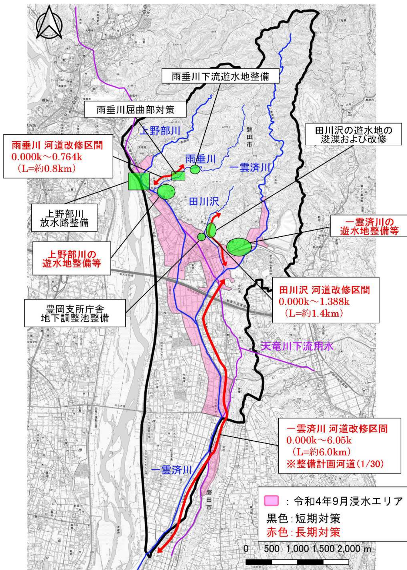
図 5.5 長期対策の整備メニュー
