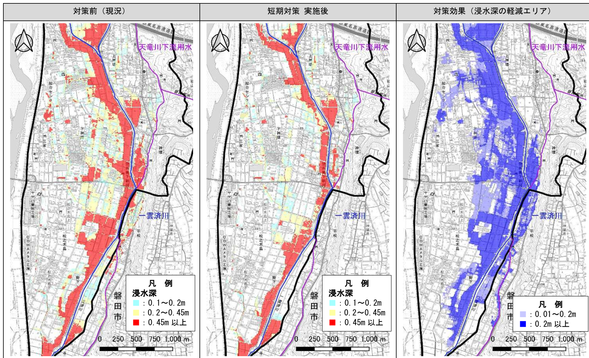
図 5.13 河川対策と流域対策によるシミュレーション結果（短期対策：合流点下流）
