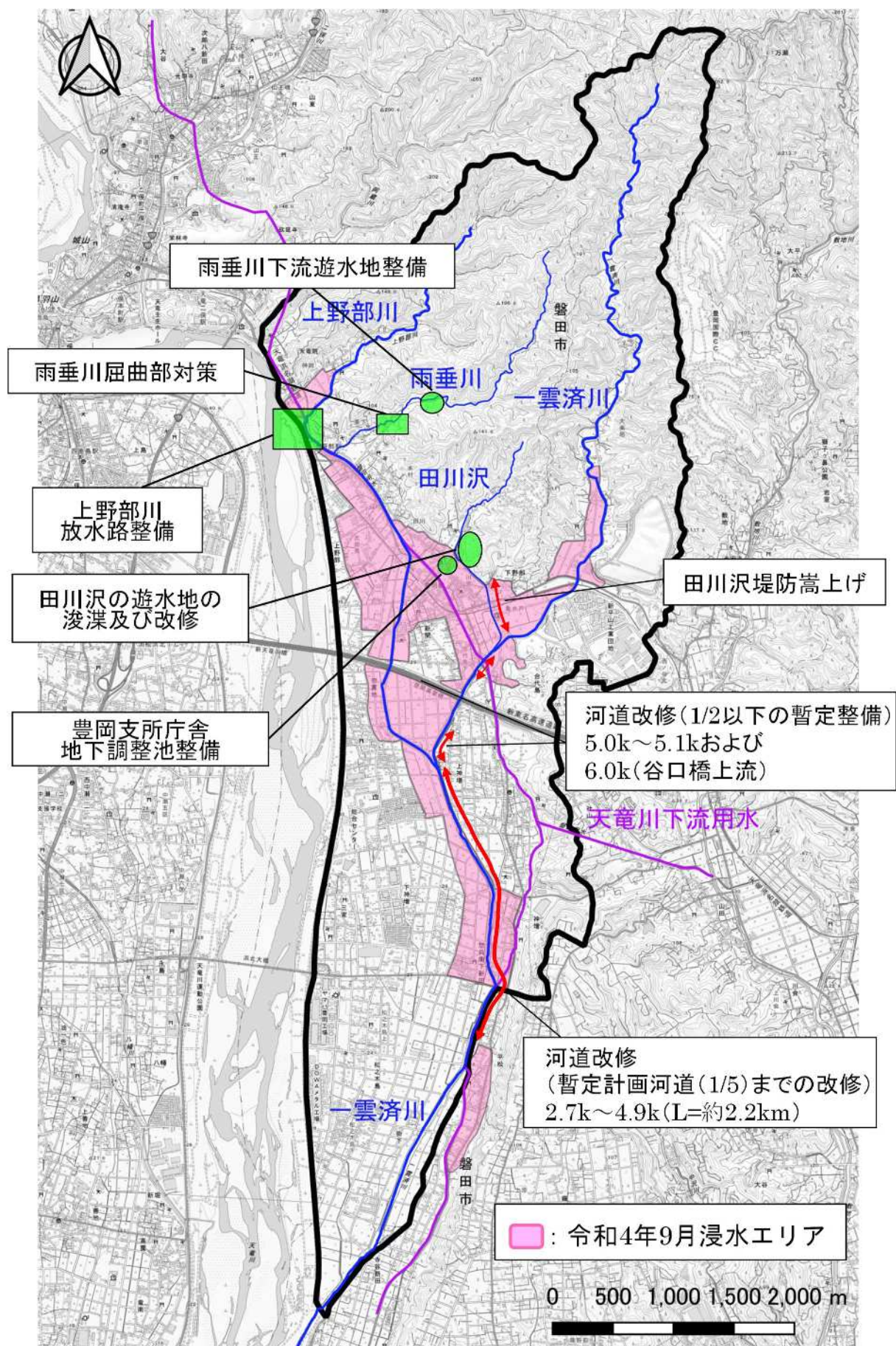
図 5.10 短期対策の整備メニュー
