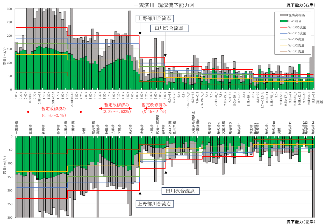
図 3.2 流下能力図（一雲済川）
