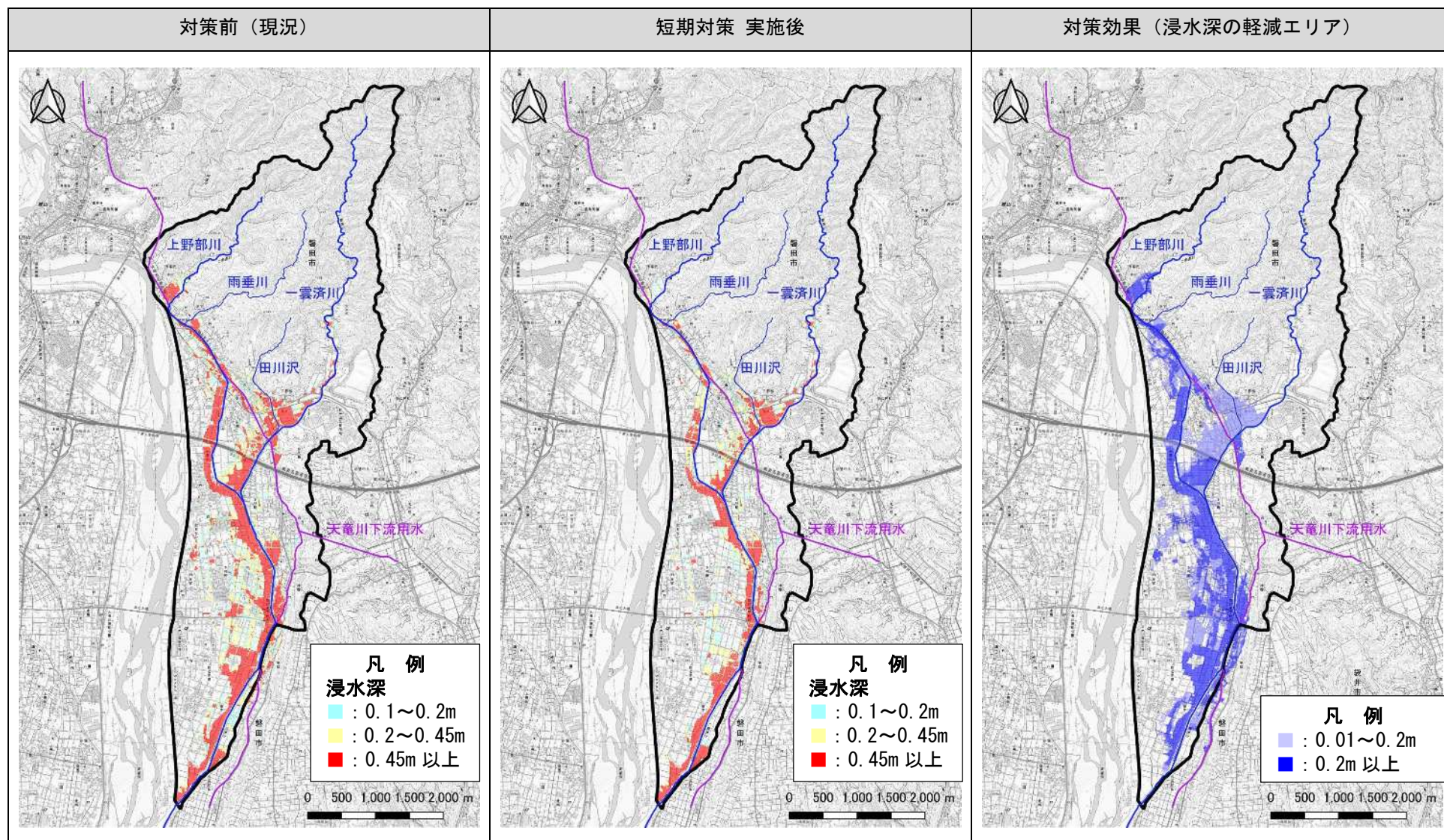
図 5.11 河川対策と流域対策によるシミュレーション結果（短期対策）
